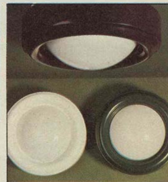
BELLMAN. Plafond i två storlekar. Lackerad metallskärm i brun, grön eller vit färg. Opalvitt acrylkupa. För många utrymmen därhemma. Form: Lennart Centervall. Plafond Bellman 1. 38 cm i diameter. Höjd från taket 14 cm. 2 ljuspunkter. Vikt 2 kg. Kr ..... 59:– Plafond Bellman 2. 25 cm i diameter. Höjd från taket 13 cm. För fast montage. Vikt 1,2 kg. Kr ..... 46:–
